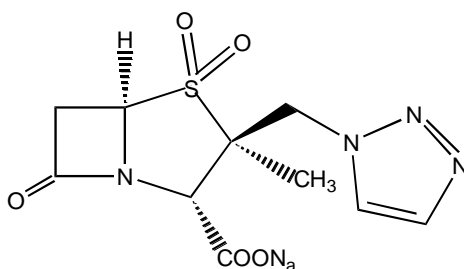
Tazobactam sodium
